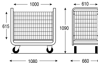
Ref. 4 444 97 03 4 Seiten (1/2 Klappe vorne) Stangenboden
