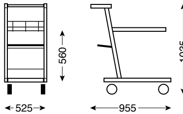
Ref. 4 461 85 03 Gewicht: 24 kg
