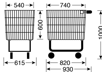
Ref. 4 461 68 03 Gewicht: 27 kg
