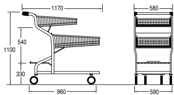
Ref. 7 788 00 03 Abstand in eingeschobenem Zustand: 345 mm
