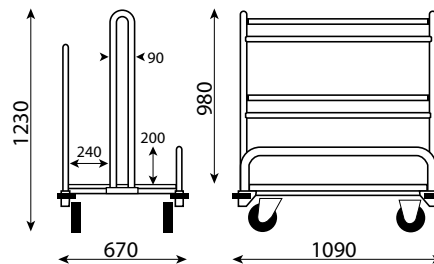
Ref. 4 447 55 03 Gewicht : 57 kg
