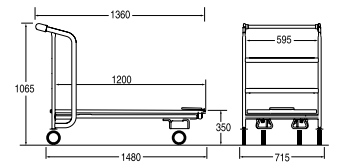
Ref. 4 459 70 03 Abstand in eingeschobenem Zustand: 340 mm Zulässige Belastung : 350 kg
