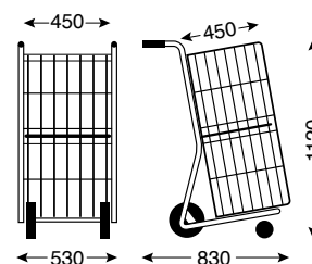
Ref. 4 461 46 03 Gewicht: 27 kg
