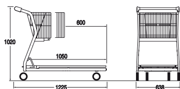
Ref. 4 454 11 03 Abstand in eingeschobenem Zustand : 352 mm Zulässige Belastung : 250 kg
