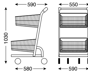
Ref. 7 788 12 03 Gewicht: 18,5 kg
