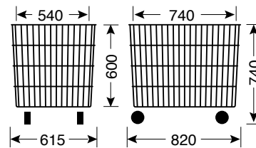
Ref. 4 461 57 03 Gewicht: 15 kg
