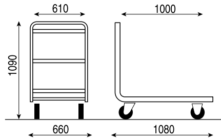
Ref. 4 444 51 03 Gekörntes Holz
